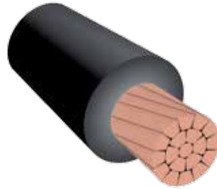
Mehrdrähtige, verdichtete Leiter
